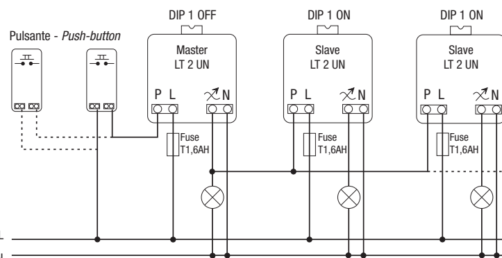
Fig. 3 - Collegamento sincronizzato - Synchronized connection
