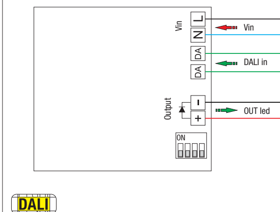
Fig. 1 - Regolazione segnale DALI 2 - DALI 2 control signal
