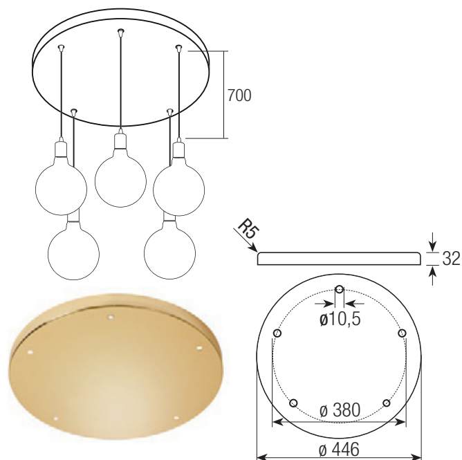
ROSONE TONDO Ø 445 - 5 FORI ROUND ROSE Ø 445 - 5 HOLES
