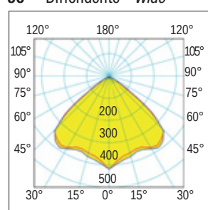
90° - Diffondente - Wide
