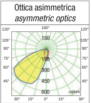
Dati fotometrici - Photometric data
